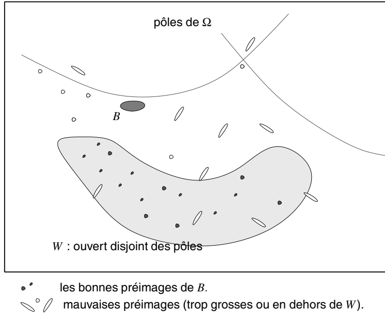
FIGURE 2. Préimages de B .
