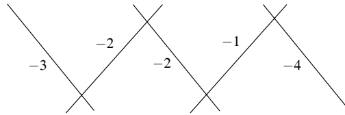
FIGURE 1. Éclatements au voisinage d'un point fixe. Diviseur obtenu après cinq éclatements. Les auto-intersections de chaque diviseur exceptionnel sont précisées.
